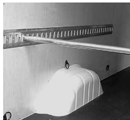
Barre télescopique
