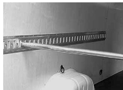
Barre télescopique
