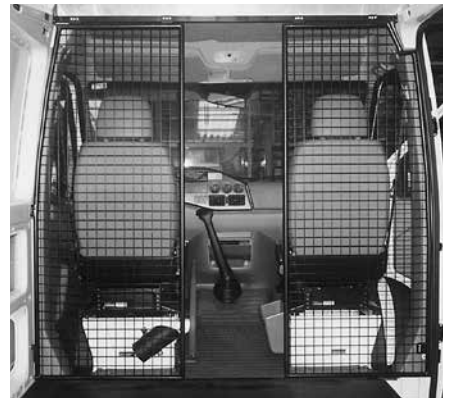
Paroi de séparation type B avec passage
